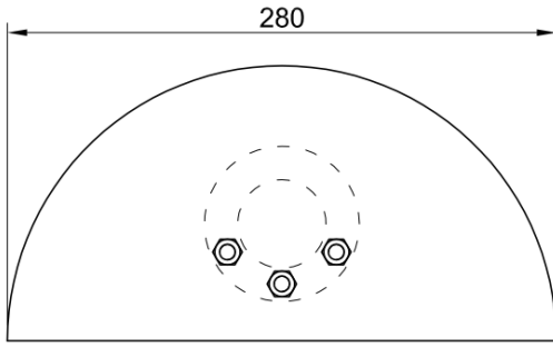
ÖNDEN GÖRÜNÜŞ
