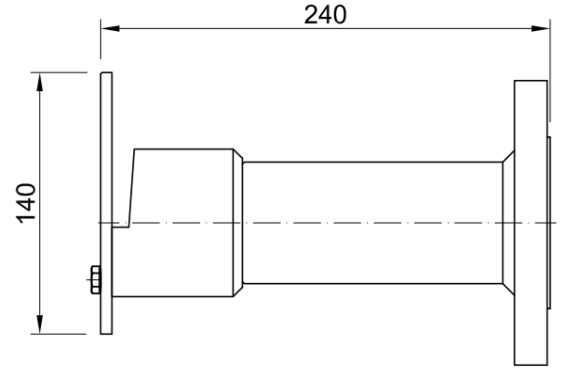
YANDAN GÖRÜNÜŞ
