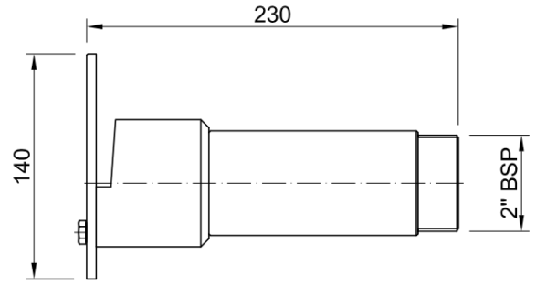
YANDAN GÖRÜNÜŞ
