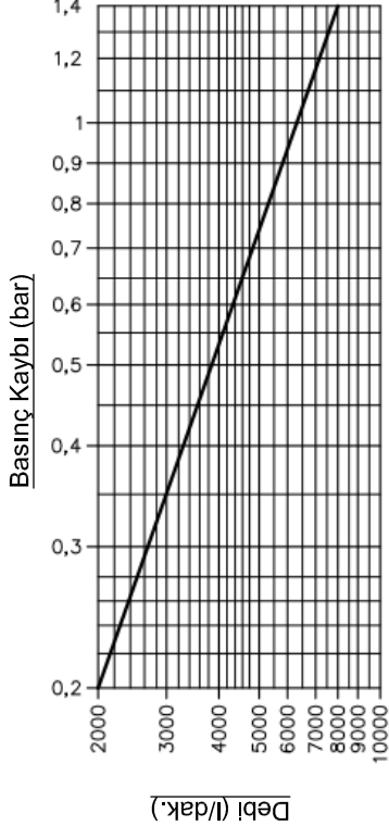
MONİTÖR BASINÇ KAYBI TABLOSU
