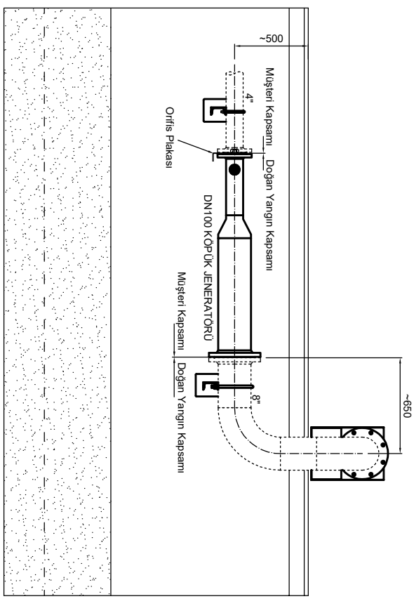
YANDAN GÖRÜNÜŞ
