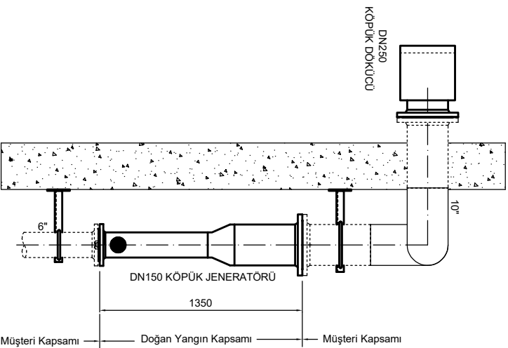
ÜSTTEN GÖRÜNÜŞ
