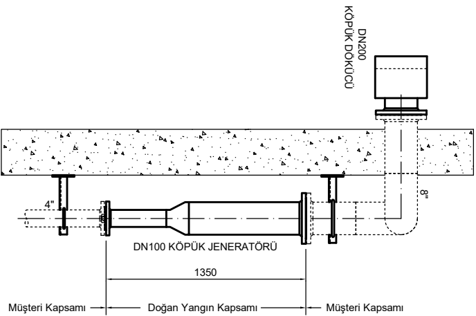
ÜSTTEN GÖRÜNÜŞ
